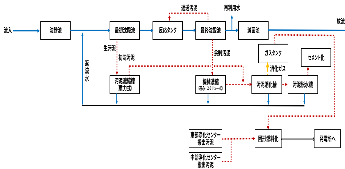
南部浄化センター処理系統図 (平成27年度末現況)
