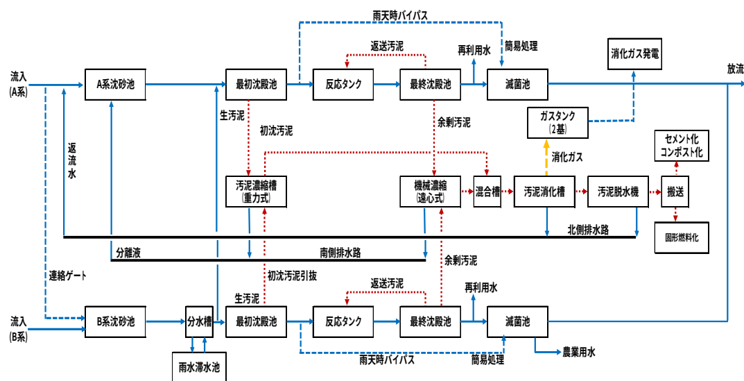
中部浄化センター処理系統図 (平成27年度末現況)
