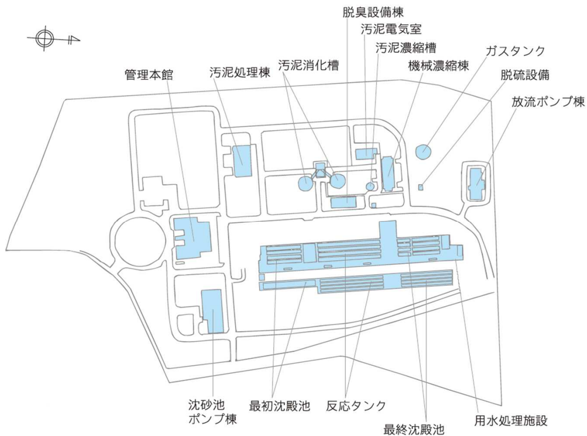
西部浄化センター処理系統図 (平成27年度末現況)
