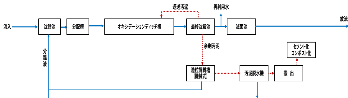
城南町浄化センター処理系統図 (平成27年度末現況)
