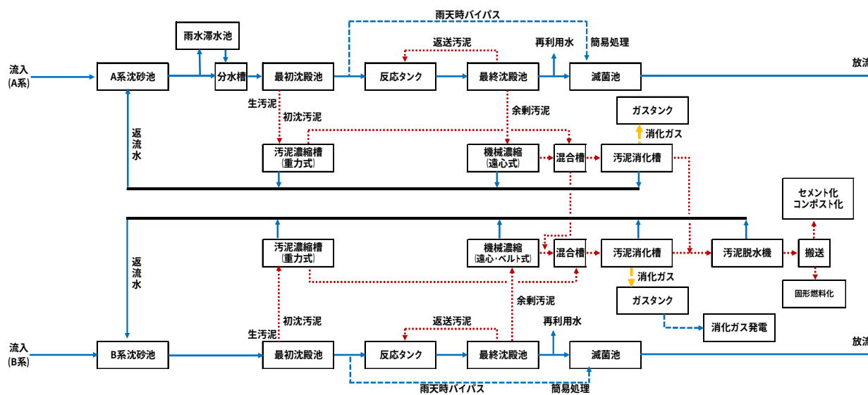
東部浄化センター処理系統図(平成27年度末現況)
