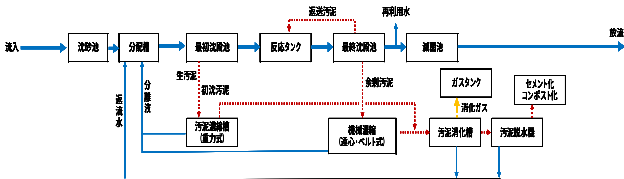
西部浄化センター処理系統図 (平成27年度末現況)
