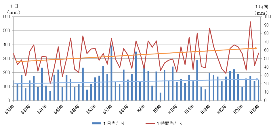
図 3-5-1-2 熊本市の最大降水量（日・時間）の推移
