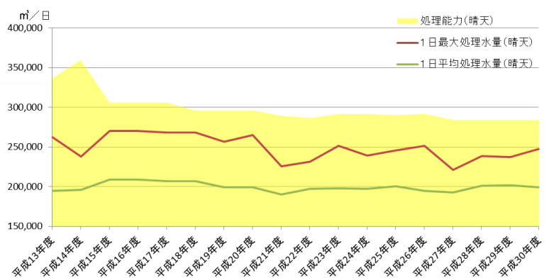
図 2-2-4 処理能力と処理量(晴天時)
