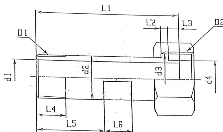
図4-2 リングユニオン \phi 13 \sim 25
