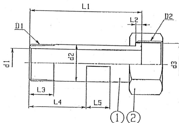
リングユニオン \phi 40
