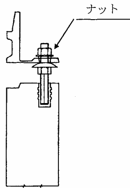
図－３ ナットによる固定
