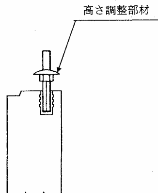
図－２ 高さ調整部材の装着
