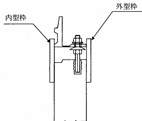
図－４ 型枠の装着
