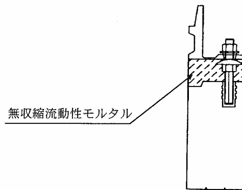
図－５ 無収縮流動性モルタルの充てん（填）
