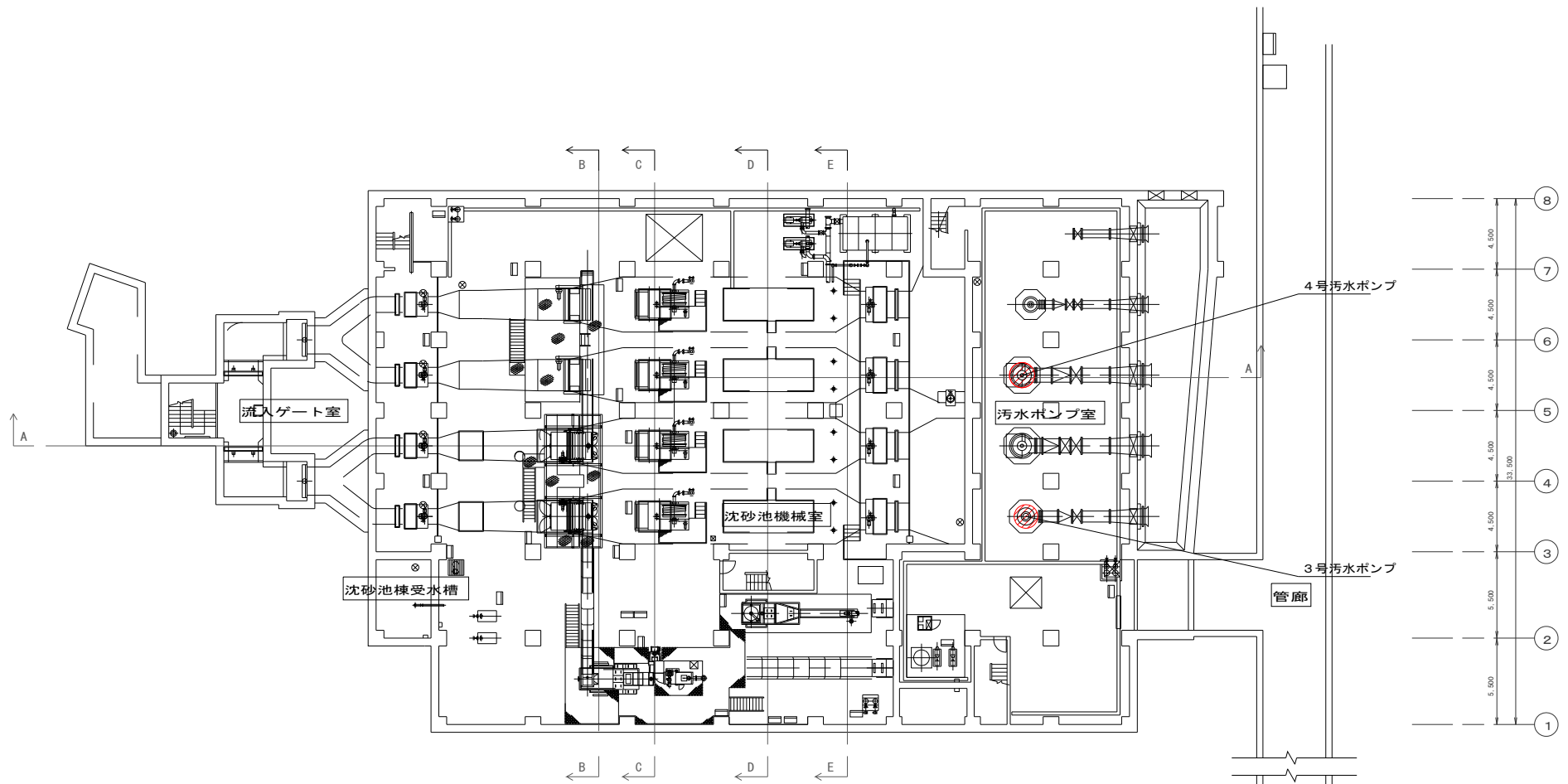
B系沈砂池設備 平面 地下1F
