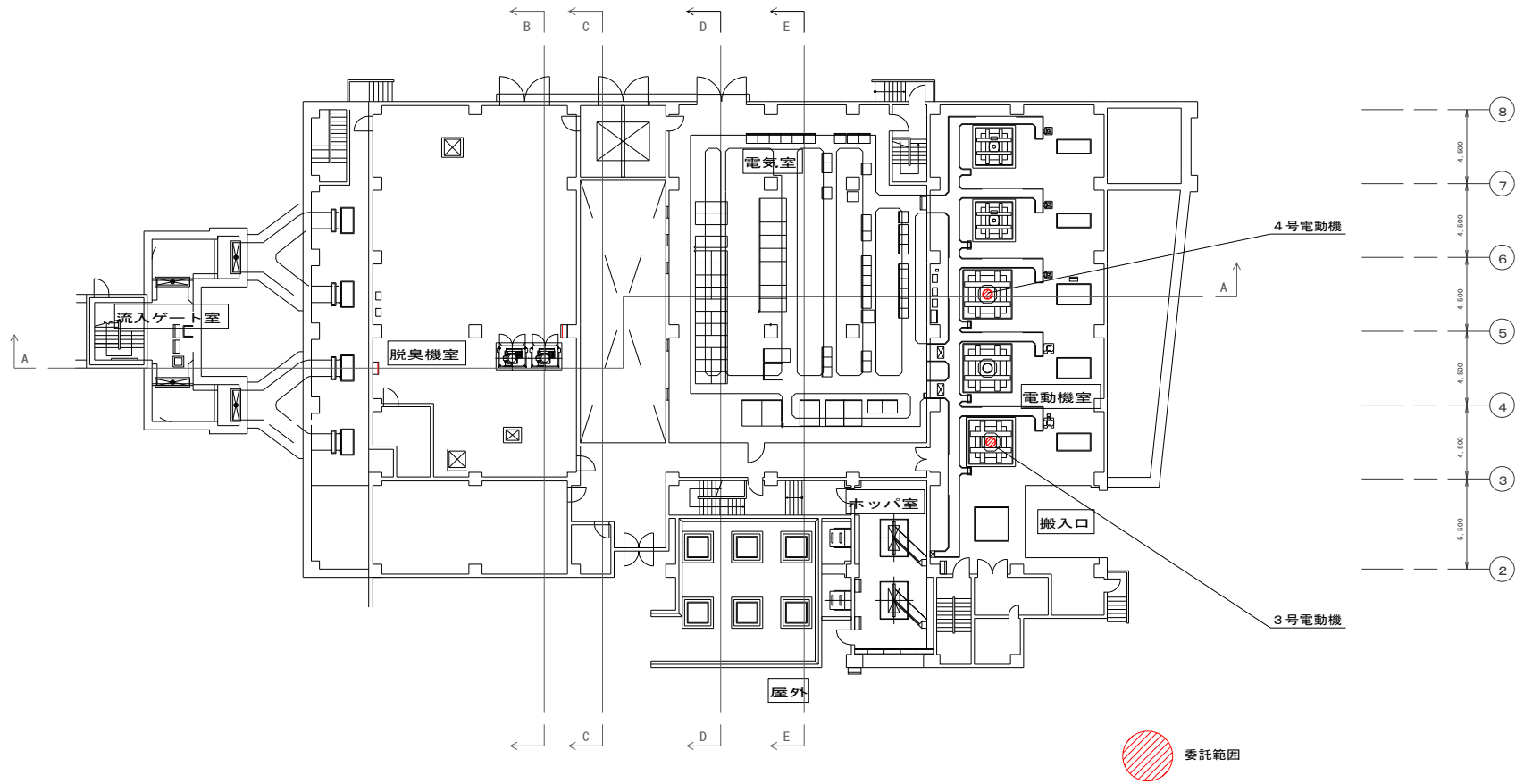
B系沈砂池設備 平面 1F
