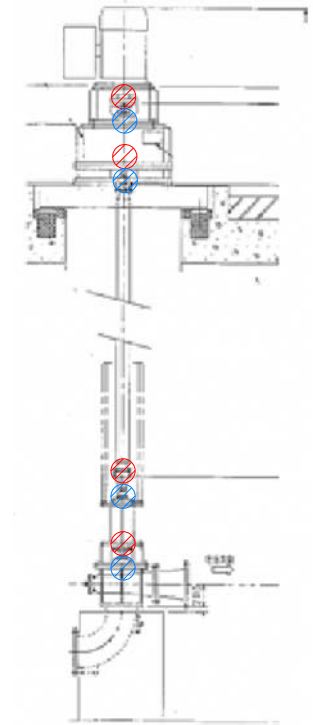
場内ポンプ場No. 1, 2号主ポンプ ポンプ側及び電動機負荷側 反負荷側潤滑油口
