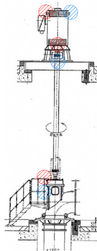
東部浄化センターB系No. 4主ポンプ 軸受ケース及び電動機負荷側反負荷側 潤滑油口
