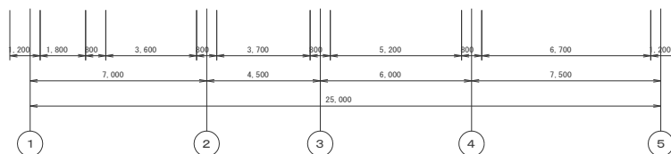
A系場内ポンプ場沈砂池設備 平面 地下2F、地下1F
