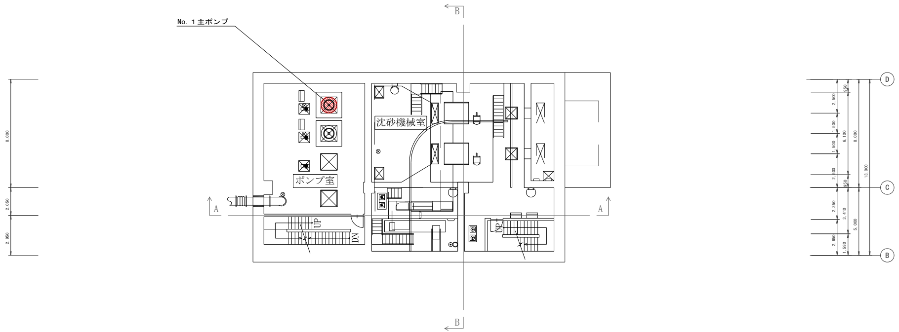
熊本市 南部 南高江ポンプ場 平面図 地下1階 200
