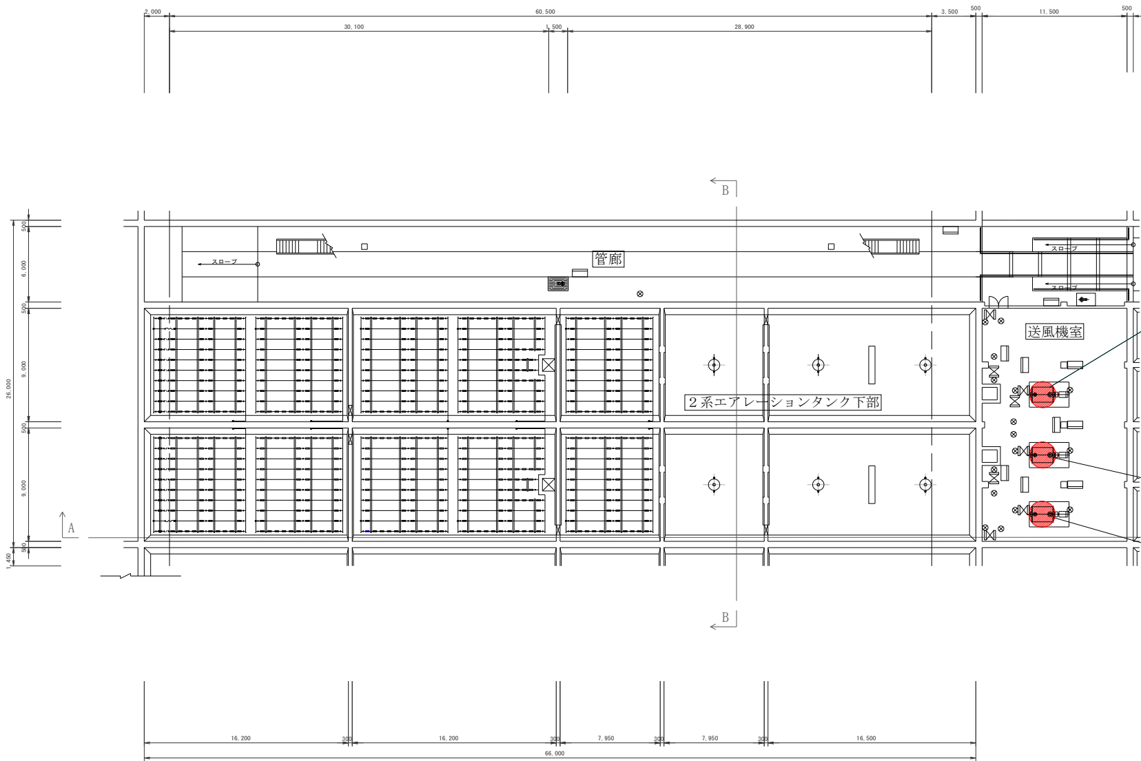
熊本市 西部浄化センター エアレーションタンク 平面地下1階
