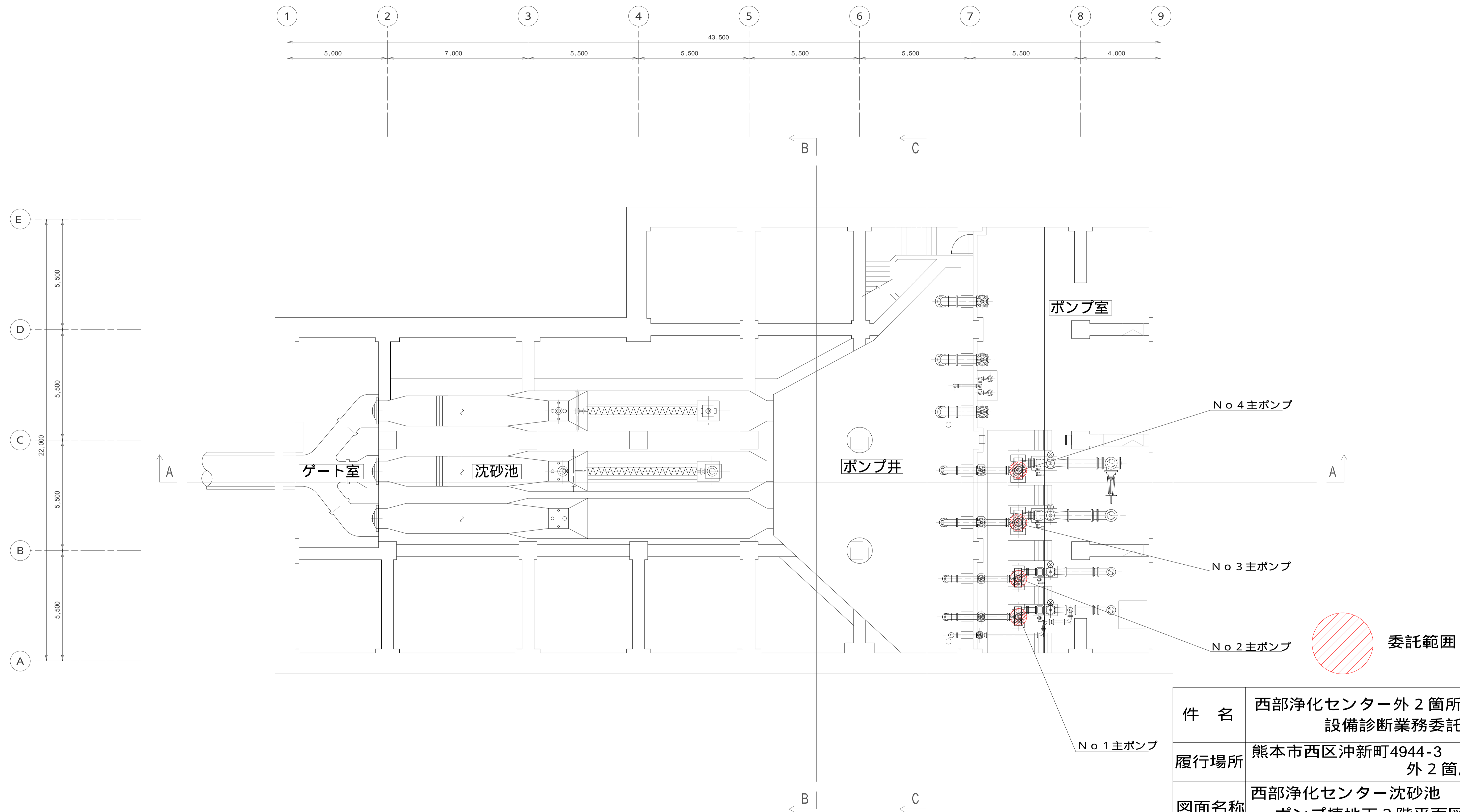
熊本市 西部浄化センター 沈砂池ポンプ棟 地下3階平面図
