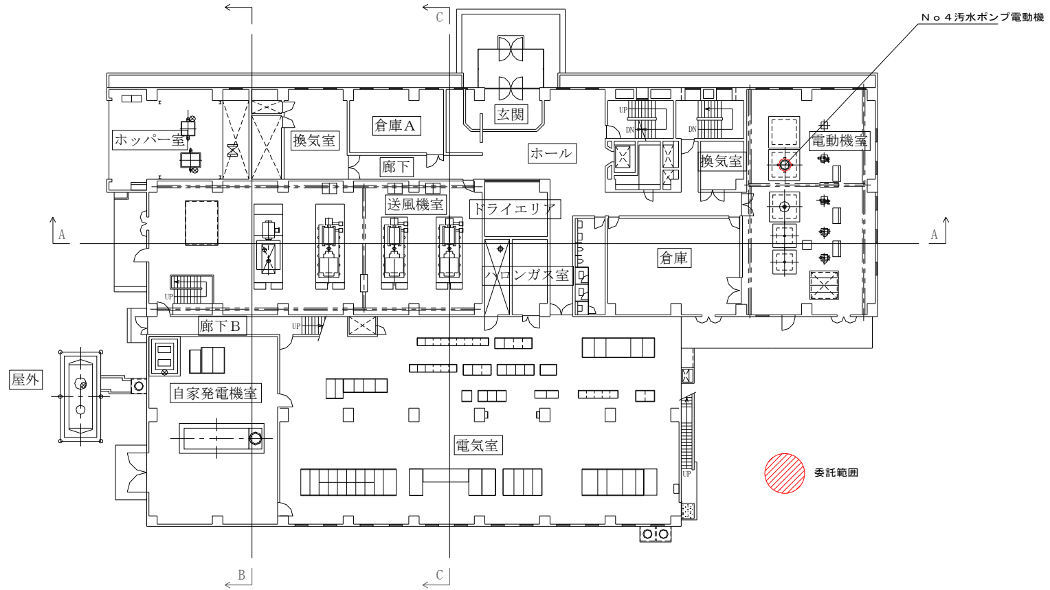
熊本市 南部浄化センター 沈砂池設備 平面 1階 300
