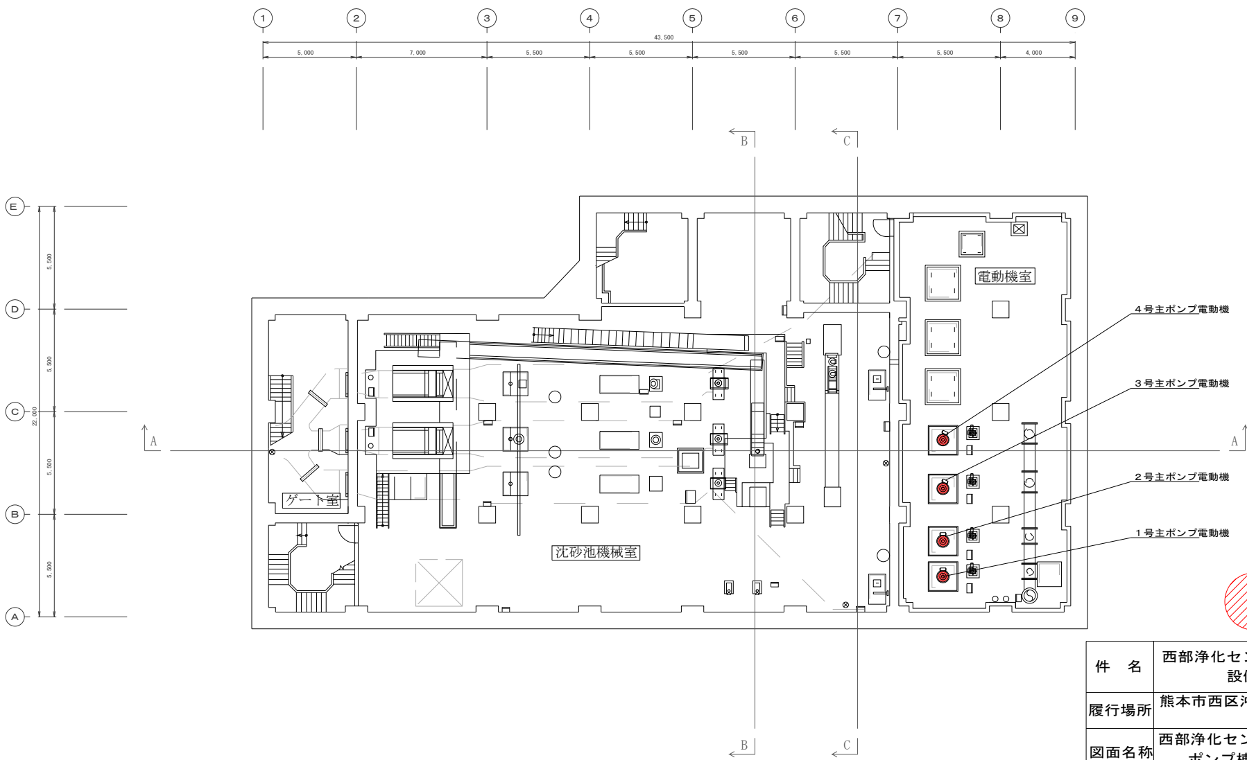
熊本市 西部浄化センター 沈砂池ポンプ棟 地下2階平面図 200
