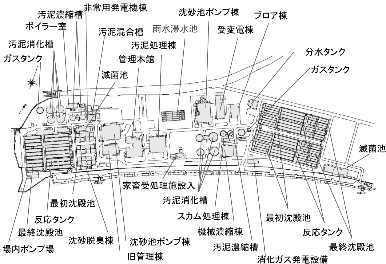
東部浄化センター処理系統図
