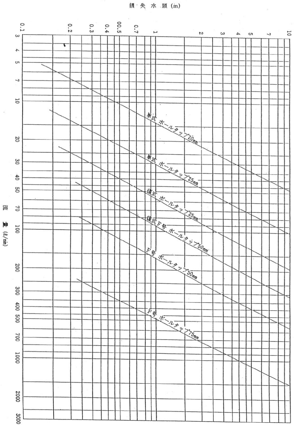
図 2-7 ホールタップ流量図表 (20~75mm)
