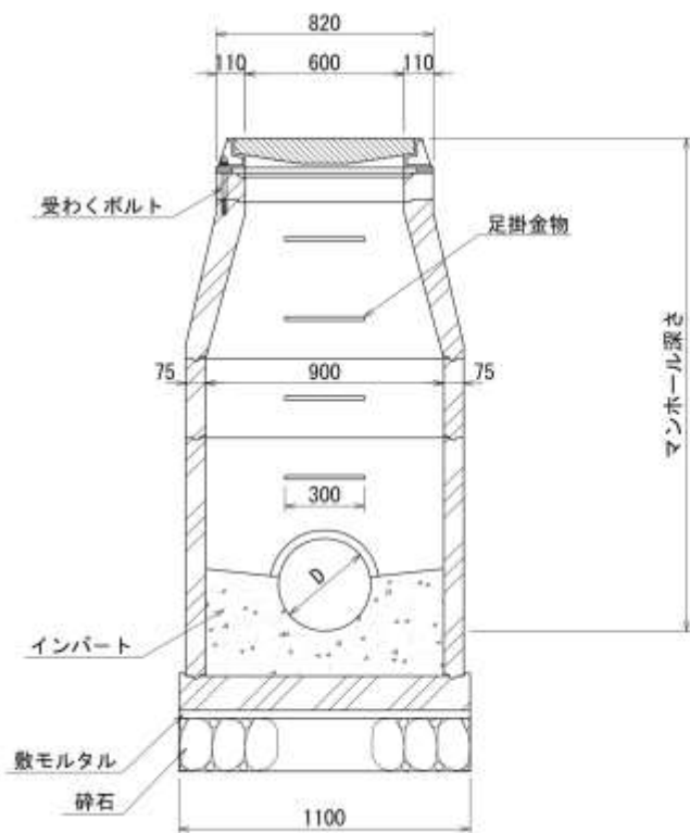
横断面図
