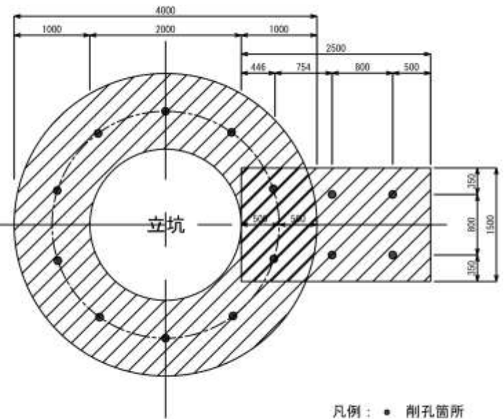
⑫改良深5.0m以下 側壁厚1.0m（坑口部1.5m×2.5m） 平面図
