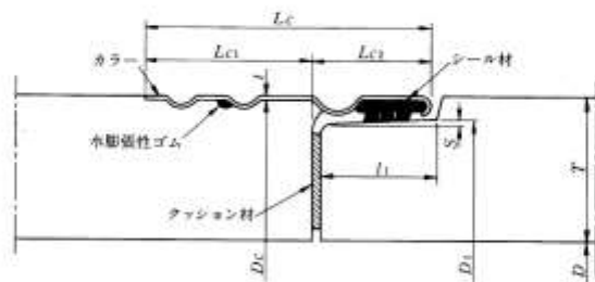
継手部詳細
