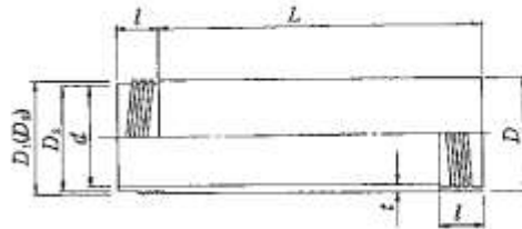
標準管
