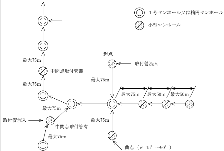
設置例
