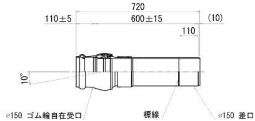
塩ビ管150mm 0° ~ 10°
