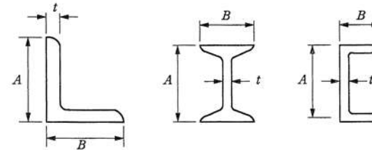
鋼材断面形状
