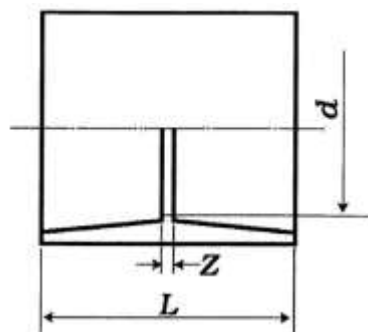
接着受ロカラー (略号 WTB)
