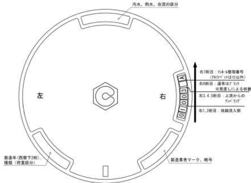
ふた表面図
