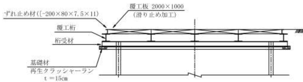
A-A 断面図
