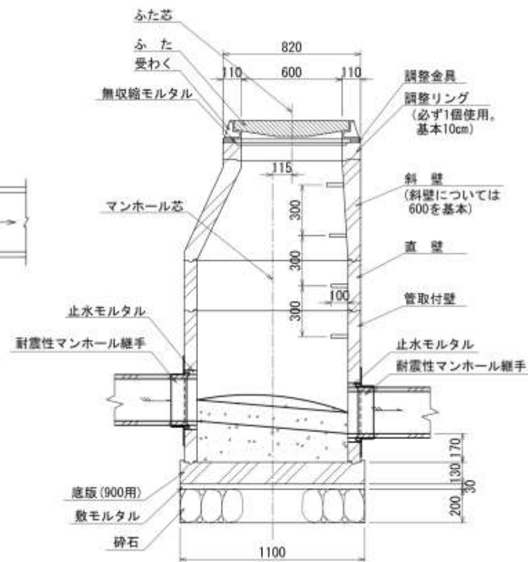
縦断面図
