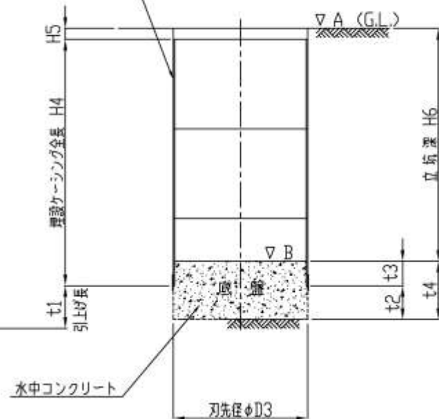
鋼製ケーシング \phi mm t mm 立坑完了図
