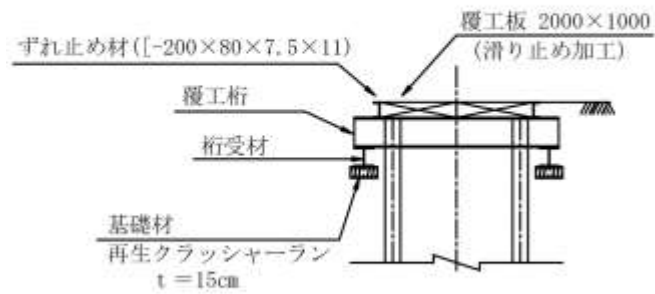
A-A 断面図
