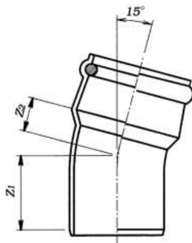
ゴム輪受口 (略号 15SR)
