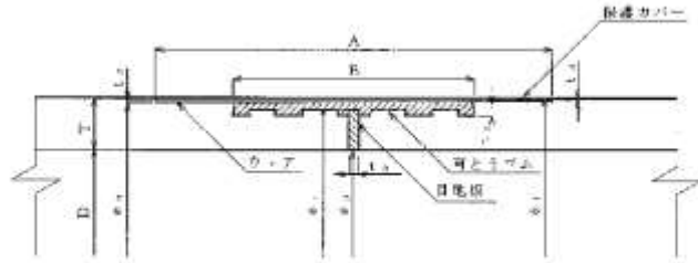
可とう部材の形状、寸法及び寸法の許容差(標準用)
