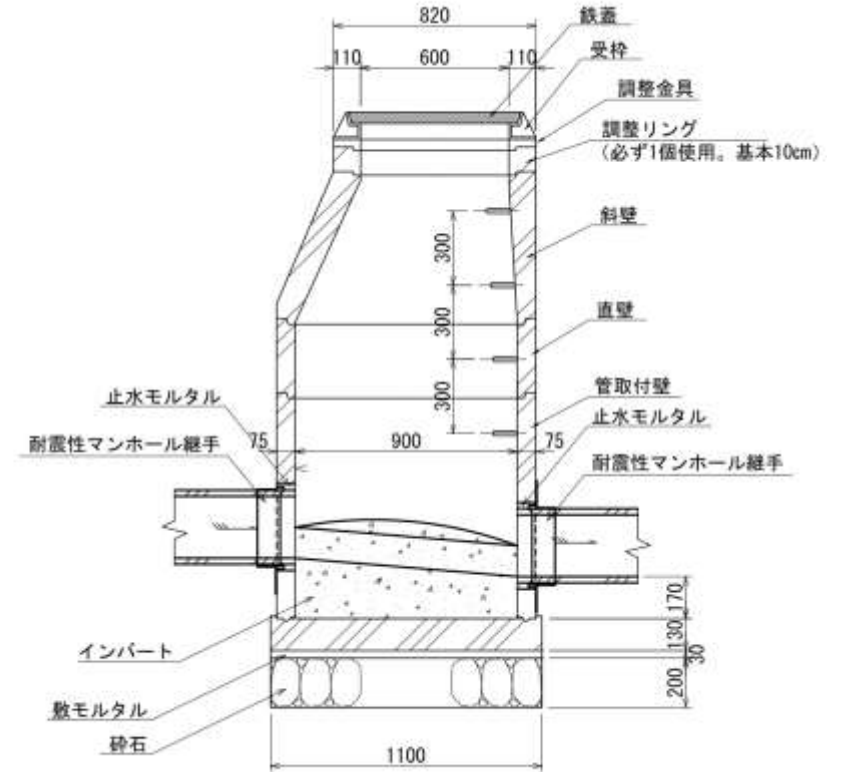
縦断面図
