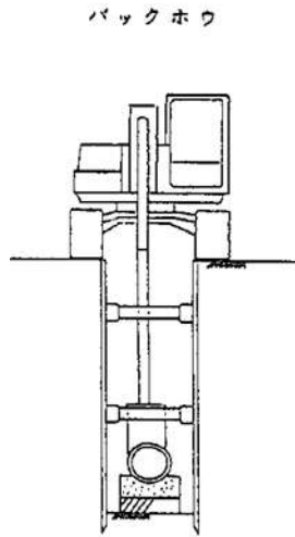
断面図
