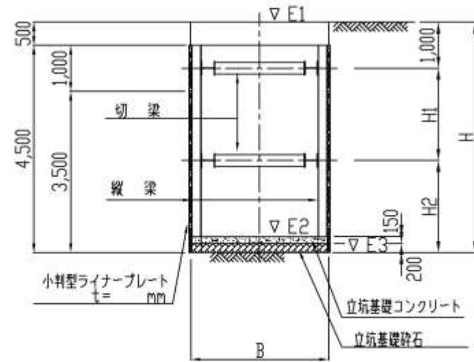
横断図
