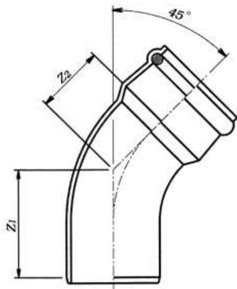
ゴム輪受口 (略号 45SR)
