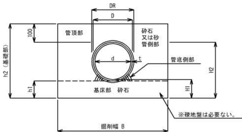
基礎寸法表
