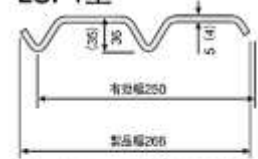
LSP1型
