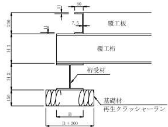
詳細図
