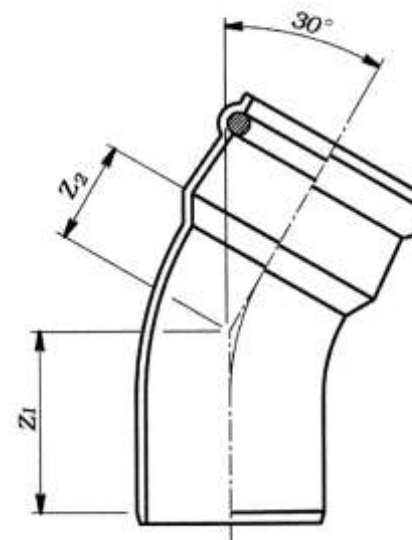
ゴム輪受口 (略号 30SR)
