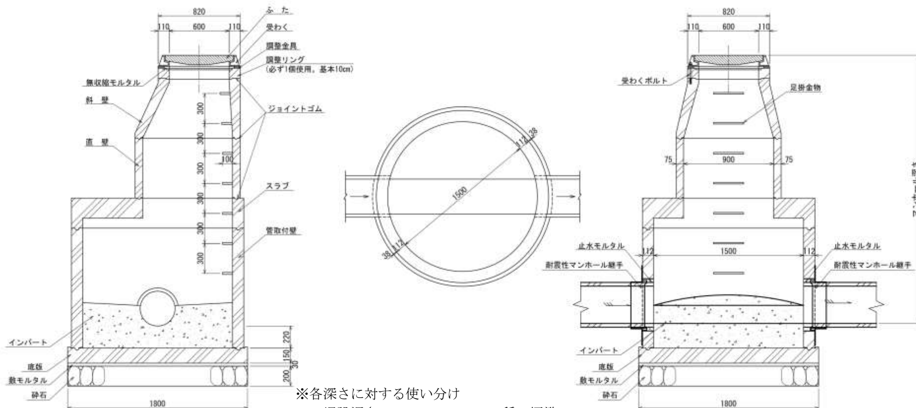
横断面図
