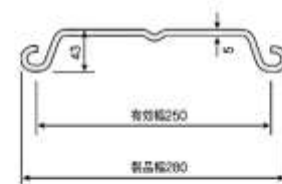
LSP2N型
