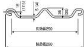
LSP2型
