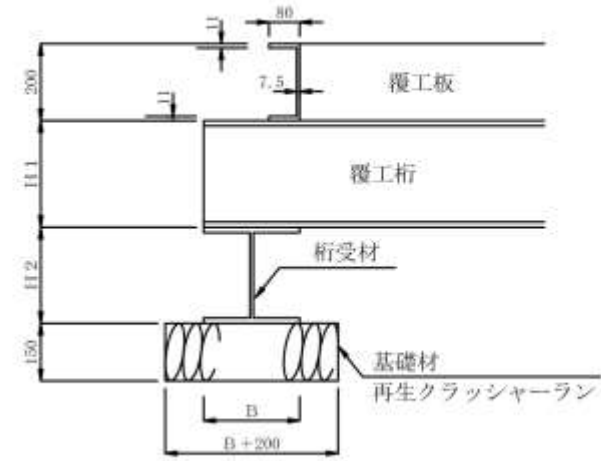
詳細図
