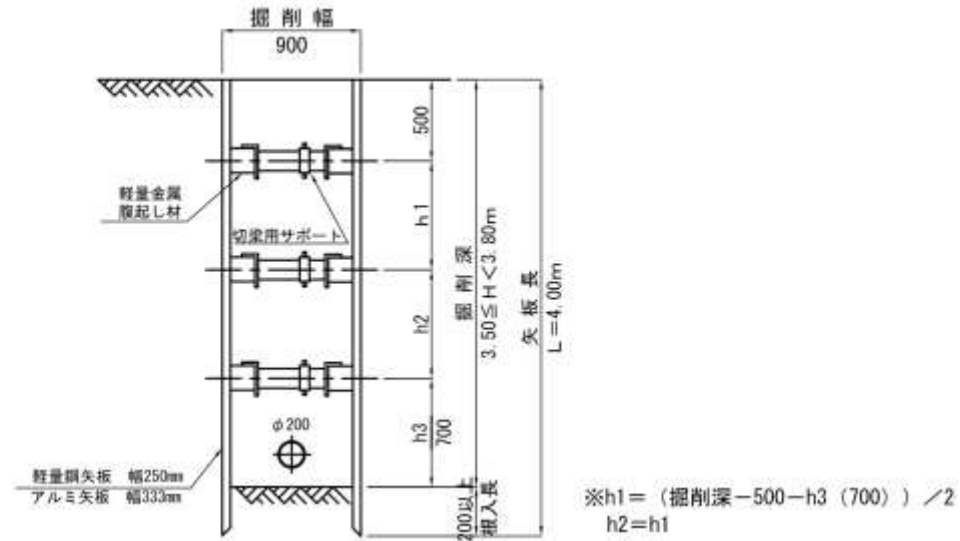
断面図 タイプ③
