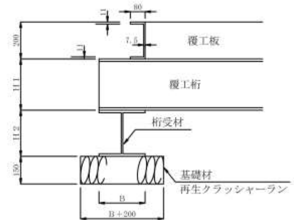
詳細図
