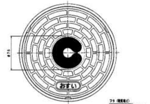
(硬質塩化ビニル製蓋)
