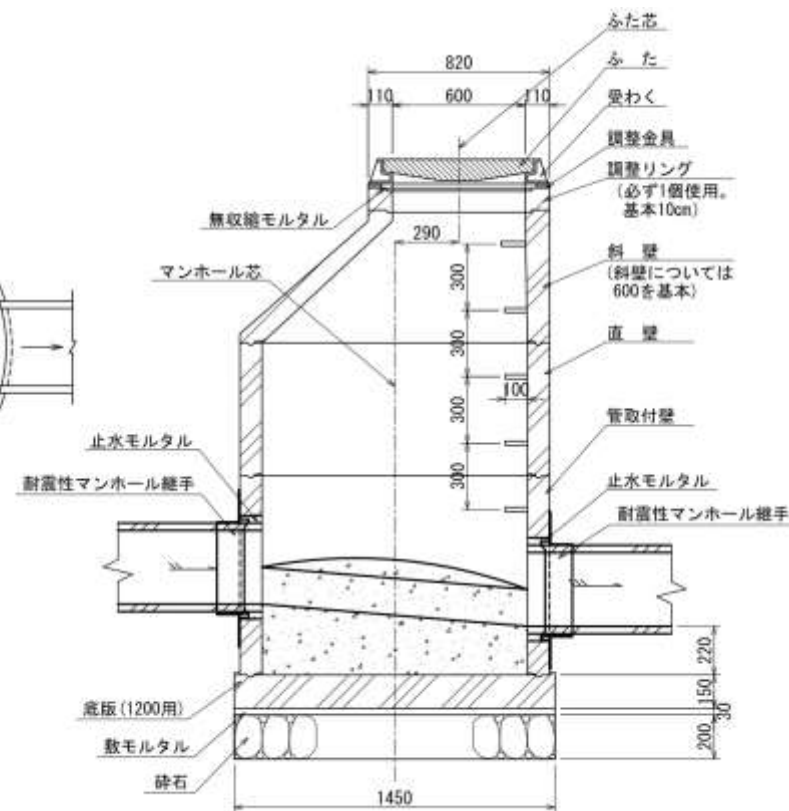
縦断面図
