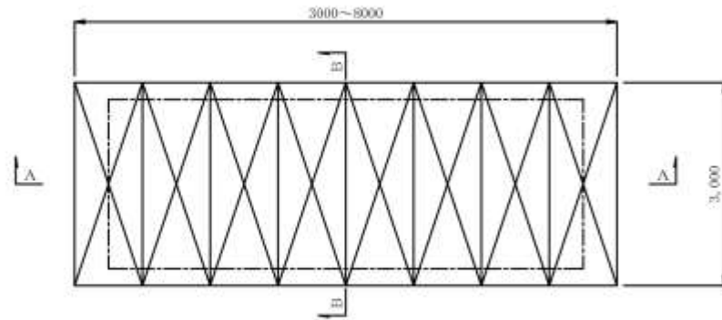
平面図
