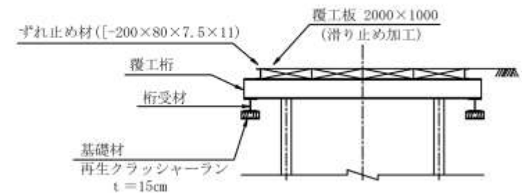
B-B 断面図
