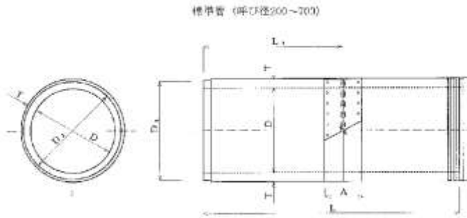
標準管の形状、寸法および寸法の許容差
