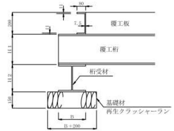
詳細図
