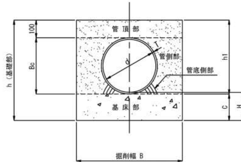
基礎寸法表
