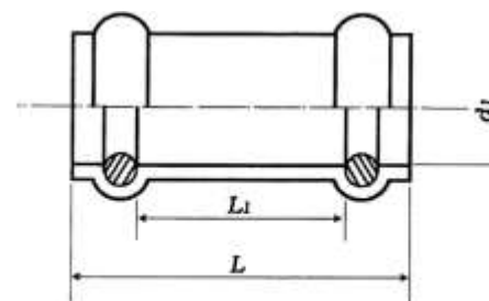
ゴム輪受ロカラー (略号 WR)
