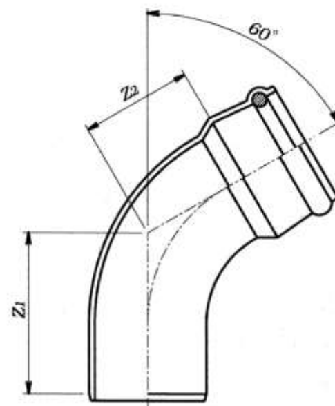
ゴム輪受口 (略号 60SR)
