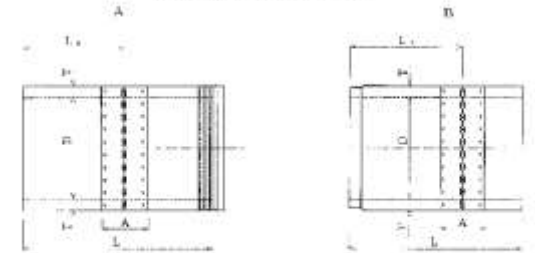
マンホール継ぎの形状、寸法および寸法の許容差 マンホール継ぎ (呼び径200~700)
