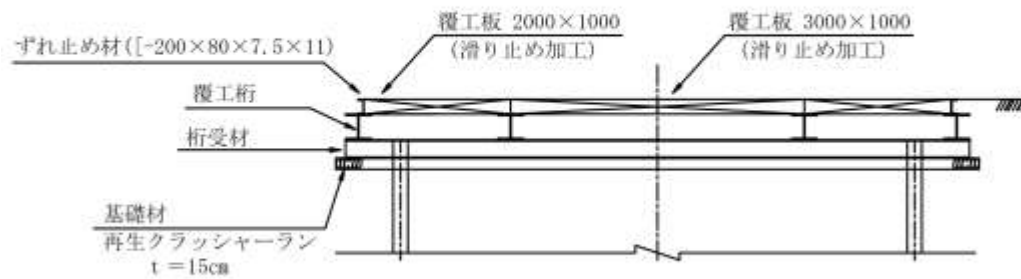
A-A 断面図
