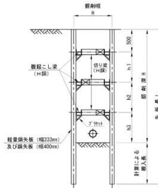
断面図
