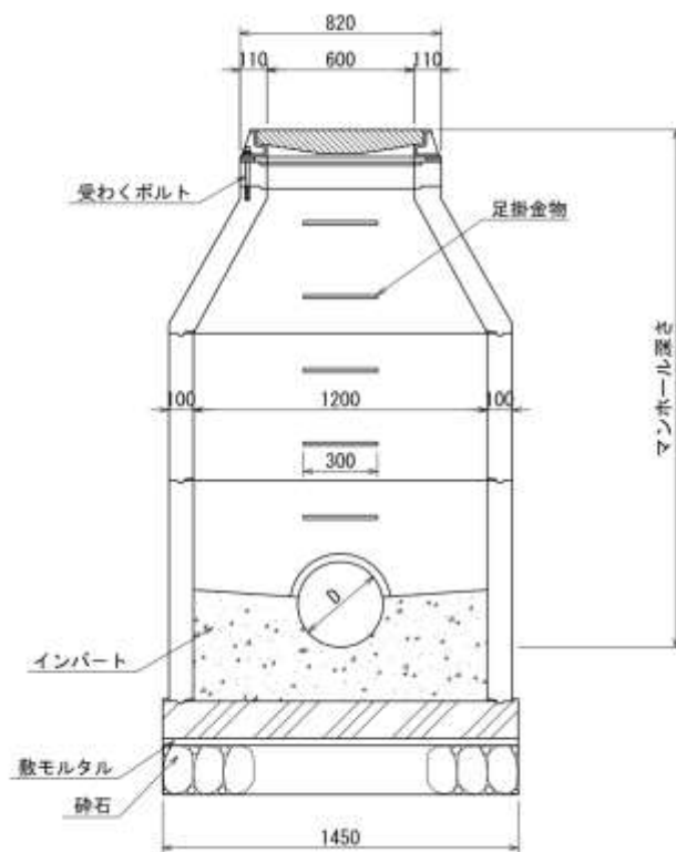
横断面図
