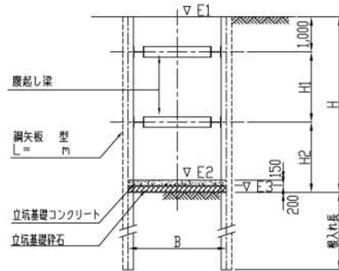
横断図
