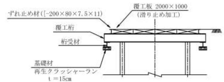
B-B 断面図
