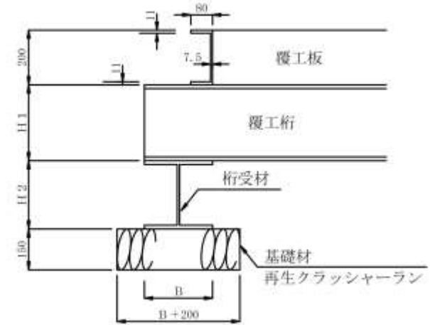
詳細図
