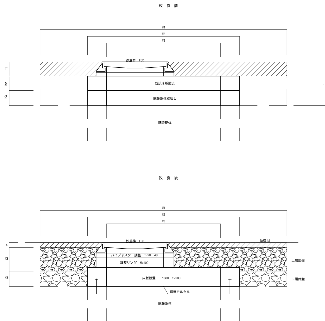
床版改良工標準断面図
