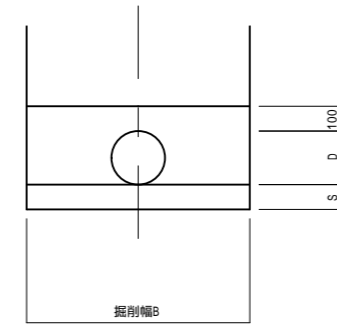
管基礎工断面図 (塩ビ管基礎)
