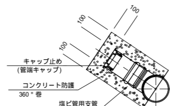
コンクリート防護断面図
