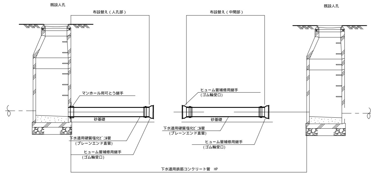
管布設工断面図 (既設管HP)
