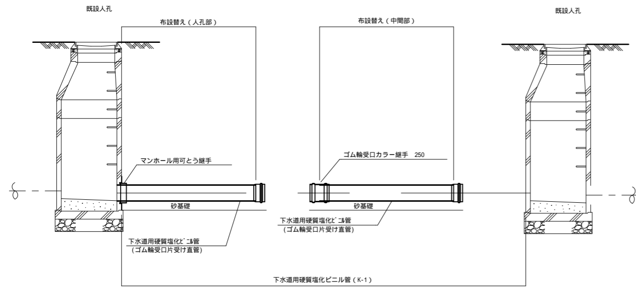
取付管閉塞工標準図
