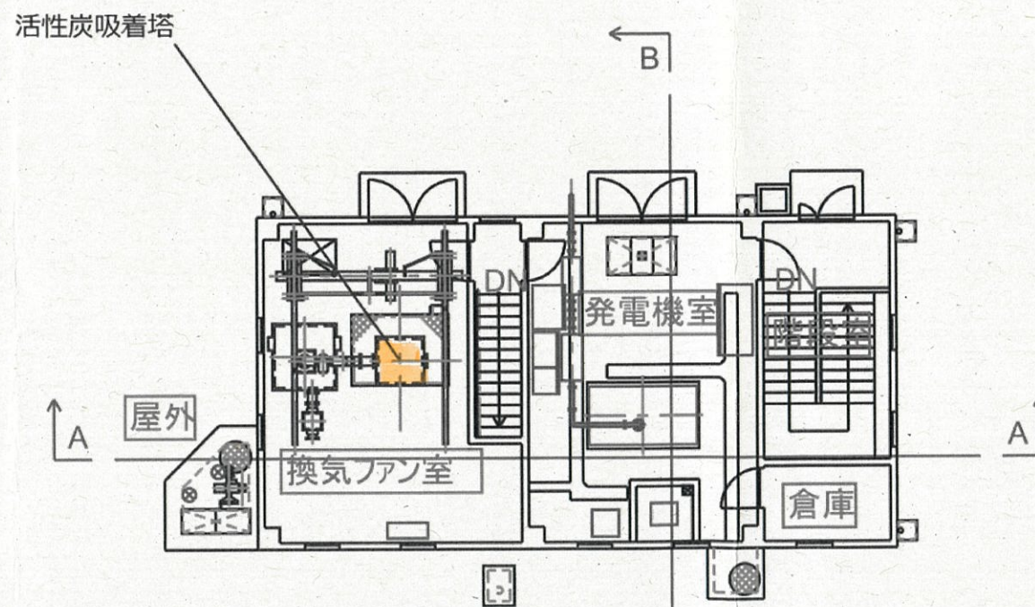
飛田ポンプ場 1階平面図
