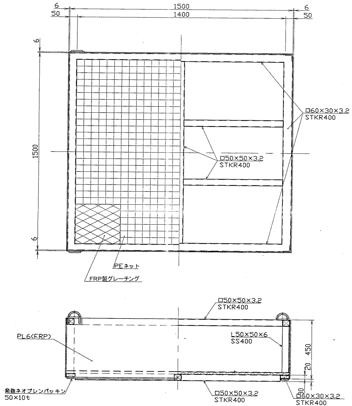
カートリッジ詳細 1/10 (充填材高さ 360) 製作数：6個
