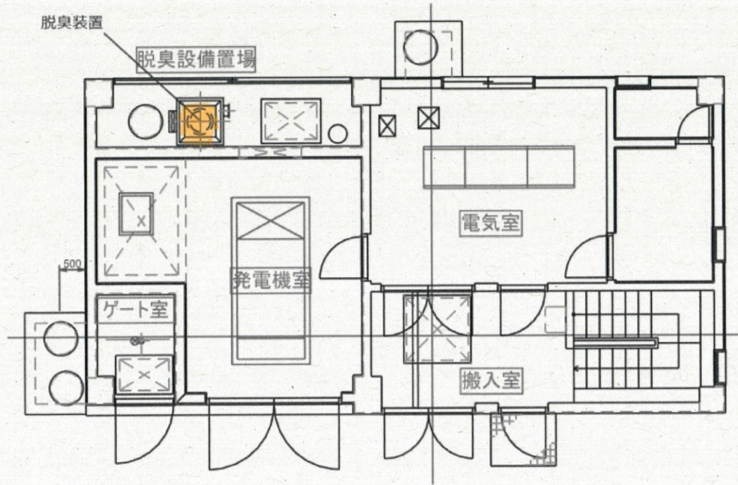
和泉ポンプ場 1階平面図
