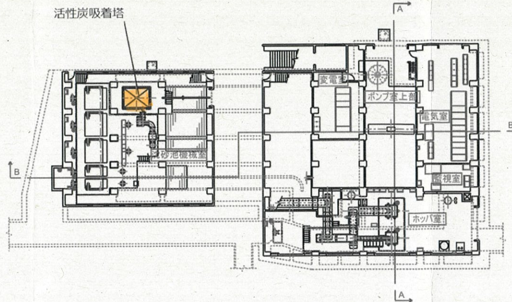
世安ポンプ場 1階平面図
