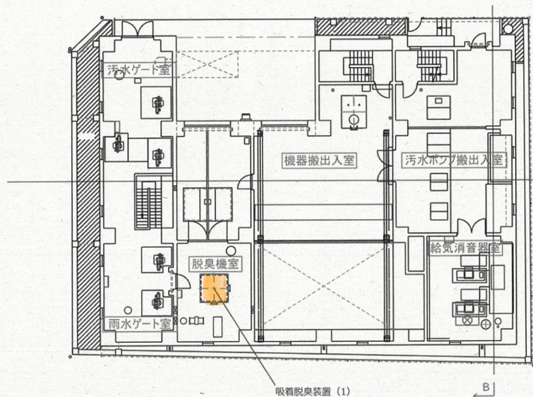
新花畑ポンプ場 1階平面図
