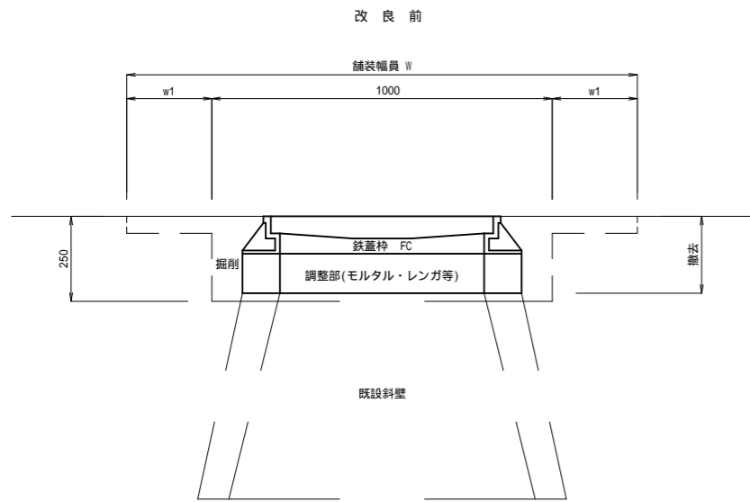
人孔改良工標準断面図
