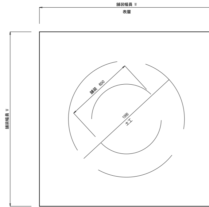
人孔改良工平面図
