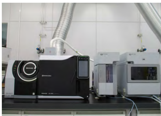
パージ・トラップガスクロマトグラフ質量分析装置 (島津製作所製GCMS-QP2020NX) (ジューエルサイエンス製PT7000)
