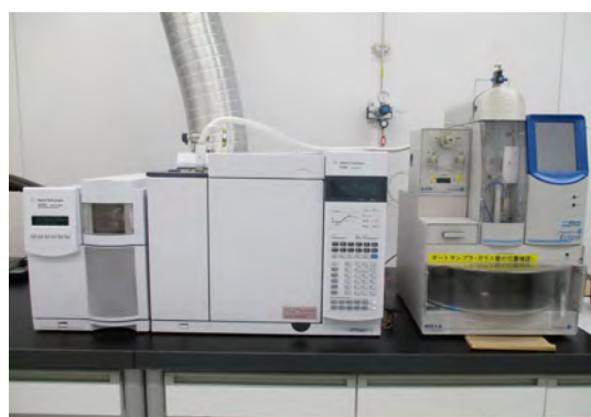
パージ・トラップガスクロマトグラフ質量分析装置 (アジレントテクノロジー製Agilent 5975C) (O・I・Analytical製Model 4660 Eclipse)
