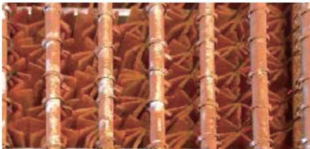
■アナモックス細菌を付着させた担体
